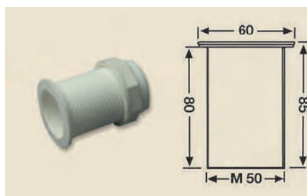
Boccola di scarico fabbricata in nylon bianco.
