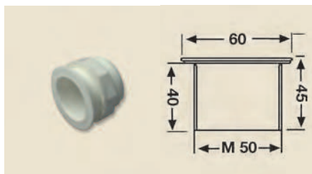
Boccola di scarico fabbricata in nylon bianco.
