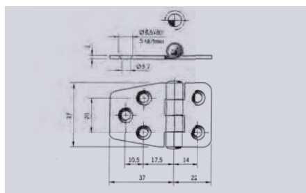
Cod. 175.60 Cerniera acciaio inox Lucidata sp. 2 mm
