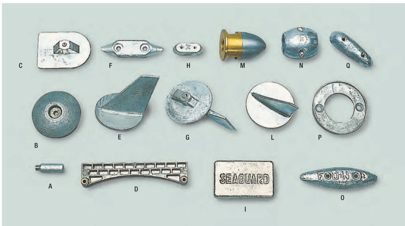
(A) Barrotto zinco filettato refrigerante motori 200 - 250 - 270.
