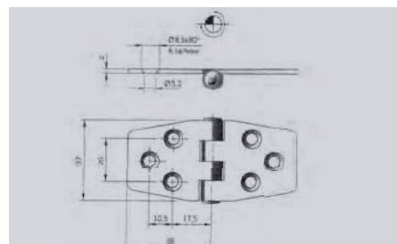
Cod. 175.59 Cerniera acciaio inox Lucidate sp. 2 mm ROVESCIAIA
