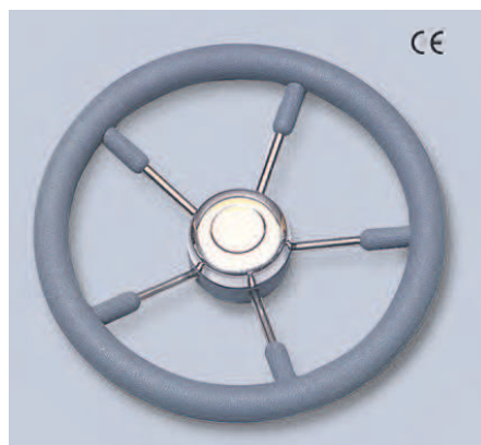
Cod. V.B 35 Ø 350 Cod. V.B 40 Ø 400 Volante inox impugnatura poliuretano colore grigio Vedi disegno C
